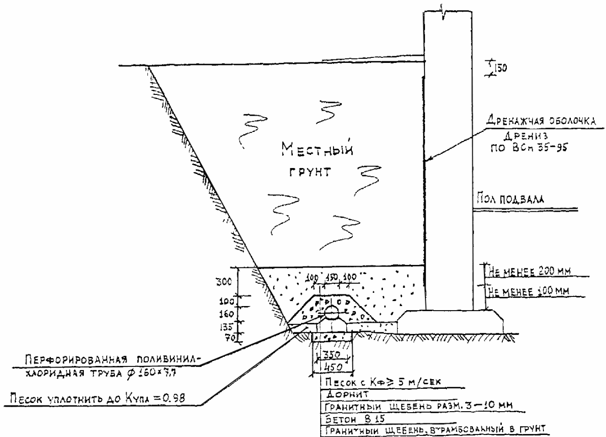
Рис. 14 Пристенный дренаж с применением поливинилхлоридных труб на бетонном основании и дренажной оболочки «Дрениз»
