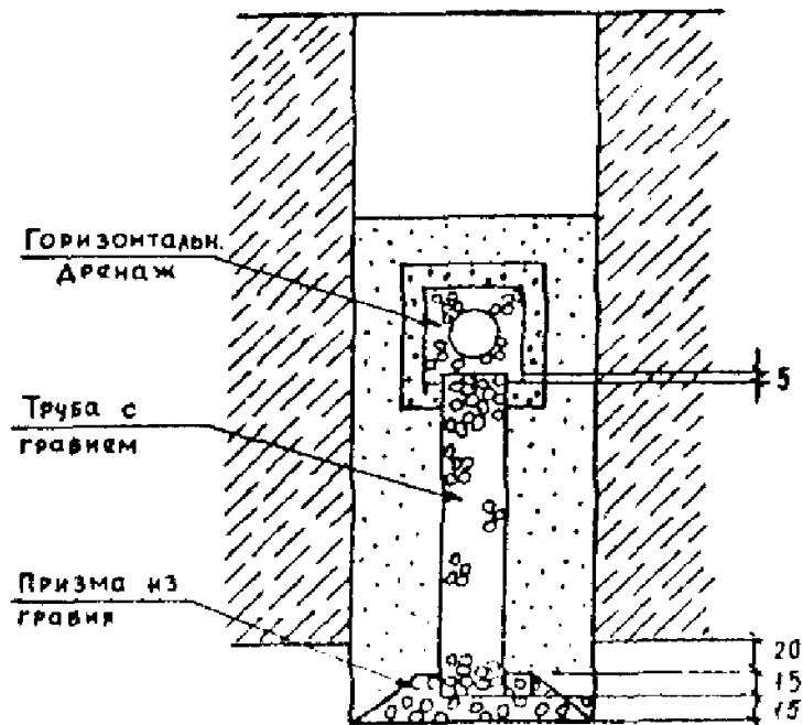
Рис. 5 Комбинированный дренаж с вертикальным самоизливающимся колодцем
