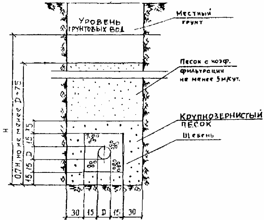
Рис. 1 Дренаж совершенного типа
