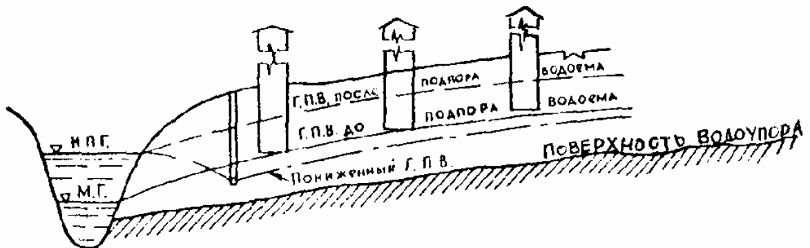
Рис. 5 Комбинированный дренаж с вертикальным самоизливающимся колодцем
